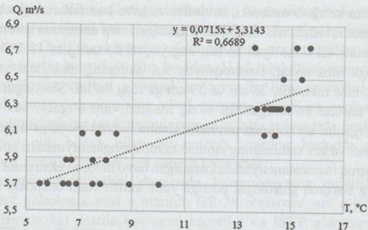
7-rasm. Barqroq meteostantsiyasida kuzatilgan havo haroratining ekstremal qiymatlari bilan Barqroq gidrologik postida o'lgan suv sarflari orasidagi bog'lanish.
