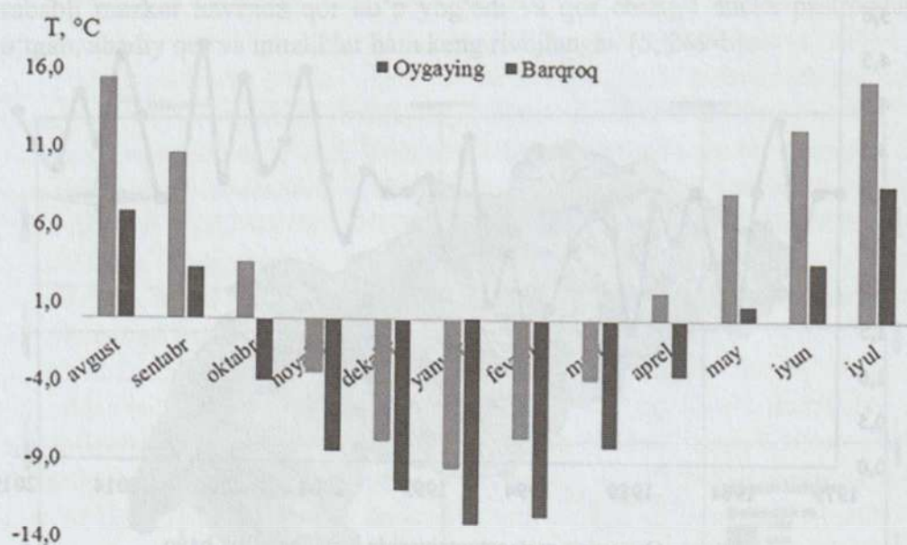
3-rasm. Oygaying va Barqroq meteostantsiyalarida qayd etilgan o‘rtacha oylik havo haroratining yil davomida taqsimlanishi.
