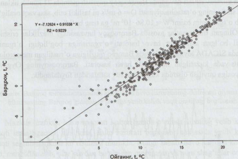
4-rasm. Barqroq va Oygaying meteorologik stansiyalarida yoz oylarida kuzatilgan o‘rtacha kunlik havo haroratlarning bog‘lanish grafiqi.
