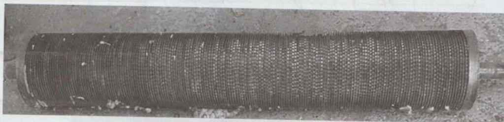
2-расм. УЧДМ русумли уруғлик чигит делинтерлаш машинасининг аррали цилиндрининг умумий кўриниши.
