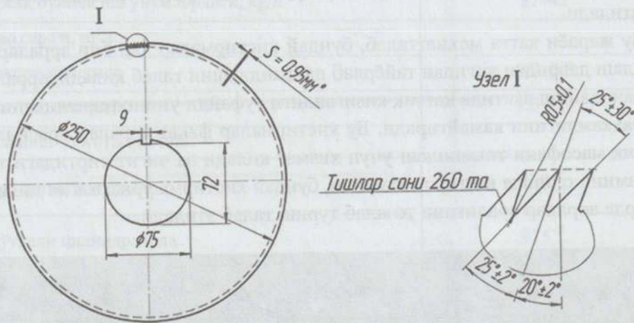
3-расм. Аррали дискнинг тиш профилнинг ўлчамлари.
