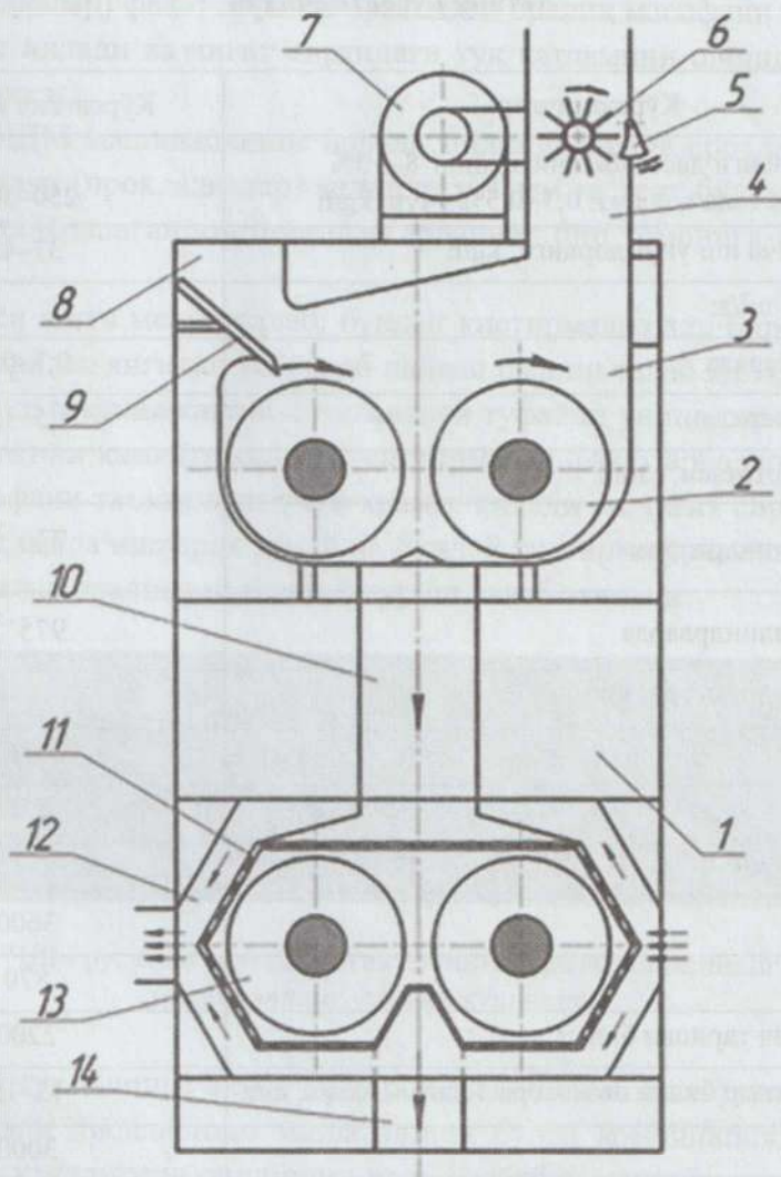
1-расм. УЧДМ русумли уруғлик чигит делинтерлаш машинасининг кўндаланг кесими схемаси.
