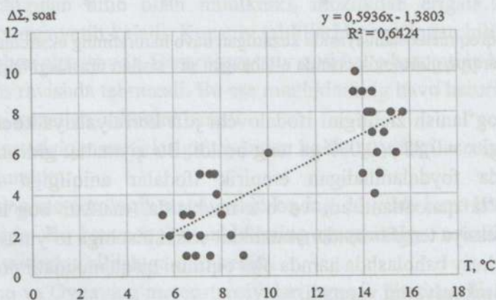
6-rasm. Barqroq meteostantsiyasida kuzatilgan havo haroratining ekstremal qiymatlari bilan suvning Barqroq gidrologik postiga yetib kelish vaqti orasidagi bog‘lanish.
