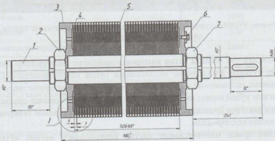
4-расм. Комбинацияланган арра-металл чўткали цилиндрининг схемаси. 1 – вал; 2 – чап ёндаги сиқувчи гайка; 3 – чап диск; 4 – арралар орасига ўрнатиладиган металл чўткали дискдан тайёрланган қистирма; 5 – арра; 6 – ўнг диск; 7 – ўнг ёндаги сиқувчи гайка.
